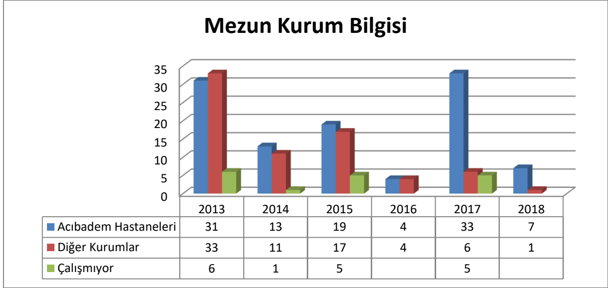
Şekil 2. Mezun Kurum Bilgisi
