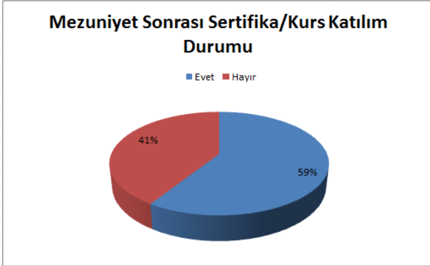
Şekil 3. Mezuniyet Sonrası Sertifika/Kurs Katılım Durumu
