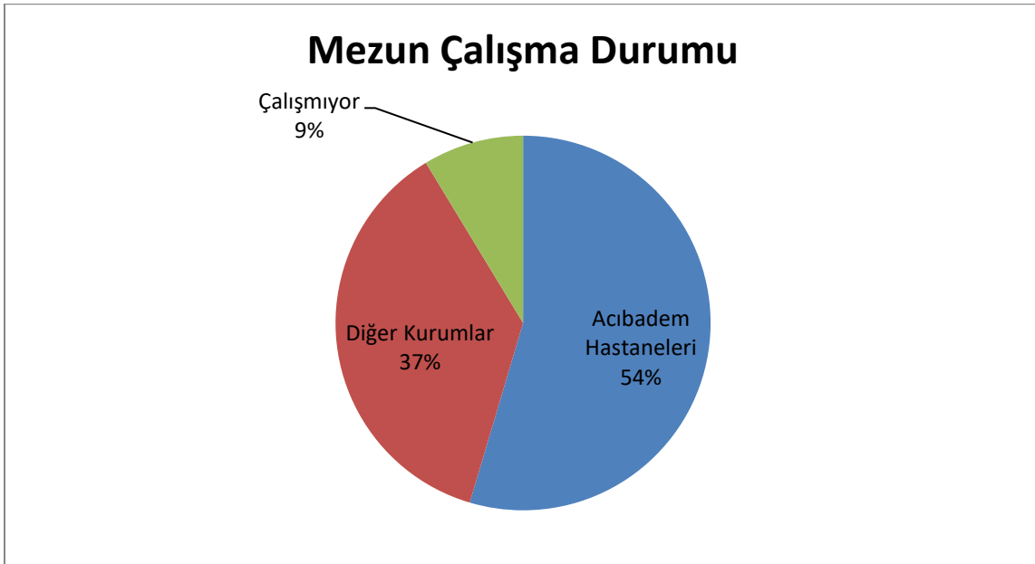
Şekil 1. Mezun Çalışma Durumu
