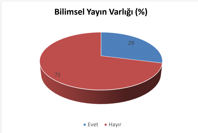
Şekil 4. Bilimsel Yayın Varlığı
